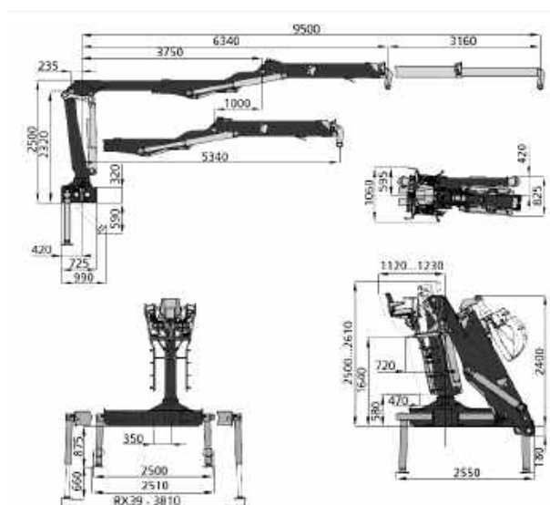
Рисунок 1. Z-подібний маніпулятор ОМТЛ-70-02
