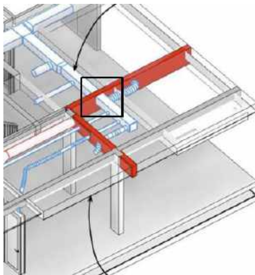
Рисунок 1. Виявлення колізій між конструкціями і інженерними мережами за допомогою BIM моделі
