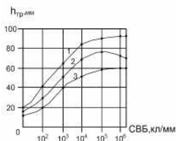
Рисунок 2. Залежності довжини тріщин в бетоні (уздовж арматурних стрижнів) від концентрації бактерій СВБ в модельному розчині. Позначення: 1 – бетон класу B40 з В/Ц=0.4; 2 – бетон класу B45 з В/Ц=0.6; 3 – бетон класу B40 з В/Ц=0.7
