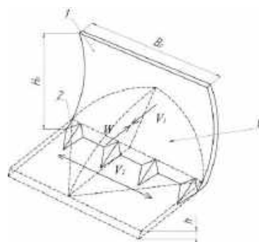
Рисунок 1. Схематичне зображення траєкторій руху робочого органу: 1 - відвал бульдозера; 2 - просторово-орієнтований ніж динамічної дії; V_1 - траєкторія руху бульдозера; V_2 - траєкторія просторово-орієнтованого ножа динамічної дії; B_0 - ширина відвалу; H_0 - висота відвалу; h - товщина шару, що зрізається
