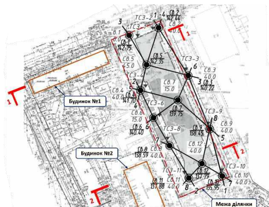
Рисунок 1. Схема розташування інженерно-геологічних виробок та розрахункових перерізів.
