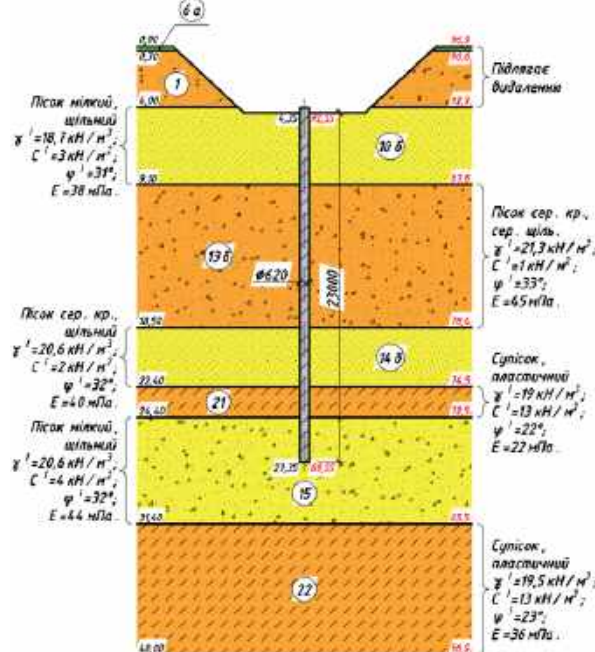
Рисунок 1. Посадка палі на геологію.
