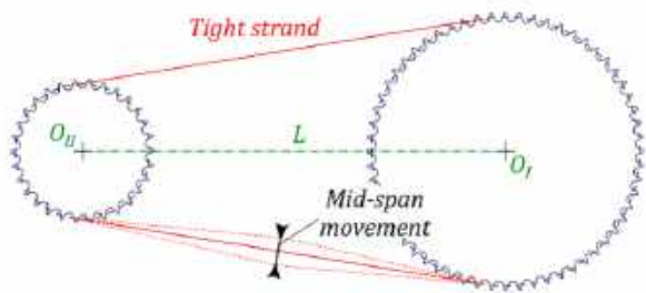
Рисунок 3. Схема провисання передачі
