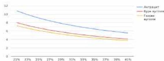
Рисунок 1. Об'єм необхідного повітря для спалювання вугілля при різних концентраціях кисню у дуттьовому повітрі, м 3 /кг
