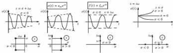
Рисунок 2. Входи, виходи і властивості передатних функцій
