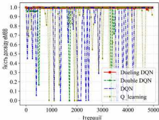
Рис. 1. Порівняльний результат якості досвіду користувачів для сервісу eMBB з різними алгоритмами
