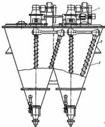
Рисунок 1. Конструкція змішувача з похилим планетарним шнековим змішувальним механізмом
