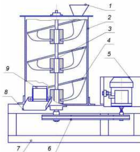
Рисунок 2. Конструкція змішувача для сухих будівельних сумішей з вертикальним валом
