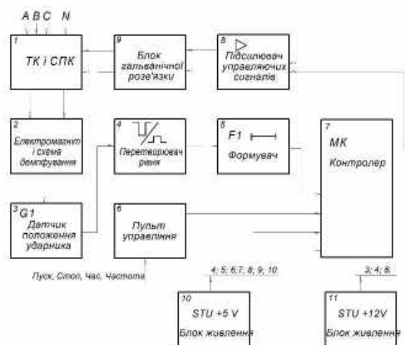
Рисунок 2. Схема функціональна блоку керування
