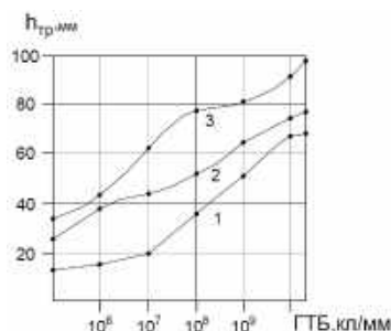
Рисунок 1. Залежності довжини тріщин в бетоні (уздовж арматурних стрижнів) від концентрації бактерій ГТБ в модельному розчині. Позначення: 1 – бетон класу B40 В/Ц=0.4; 2 – бетон класу B45 з В/Ц=0.6; 3 – бетон класу B40 з В/Ц=0.7
