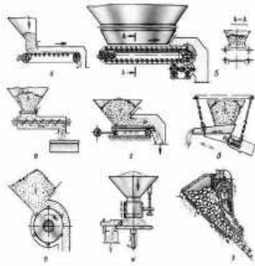
Рисунок 2. Схеми живильників: а – стрічковий; б – пластинчатий; в – гвинтовий; г – коливальний; д – вібраційний; е – барабанний; ж – дисковий; з – ланцюговий
