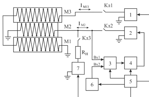
Рисунок 1. Структурна схема експериментальної установки: M1, M2, M3 – термоелектричні модулі; 1, 2 – керовані джерела імпульсного струму; 3,7 – комутатори аналогових сигналів; 4 – пристрій реєстрації; 5 – мікропроцесорна система керування; 6 – блок калібрувальних сигналів.
