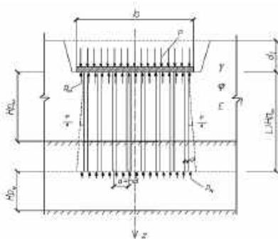
Рисунок.2 Розрахункова схема взаємодії крупнорозмірного плитно-пальового фундаменту з ґрунтовим масивом [3]
