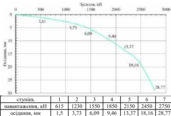
Рисунок 2. Графік випробування палі.
