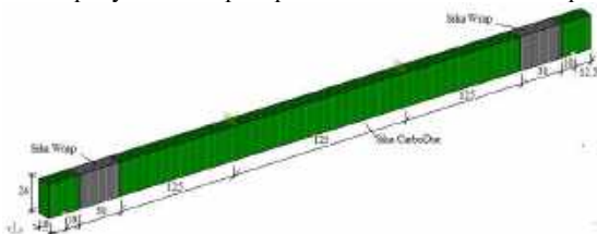
Рисунок..1 Балка з клеєної деревини підсилена композитними стрічками прольотом 4 м, змодельована в ПК ЛІРА-САПР.
