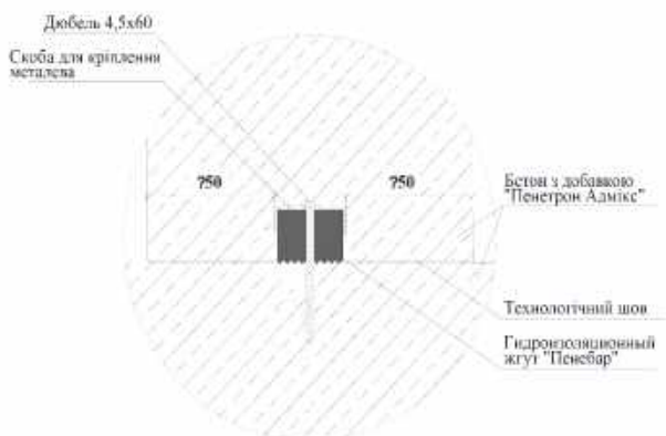
Рисунок 3. Приклад конструктивного рішення застосування гідрофільного джгута для герметизації швів у монолітних конструкціях
