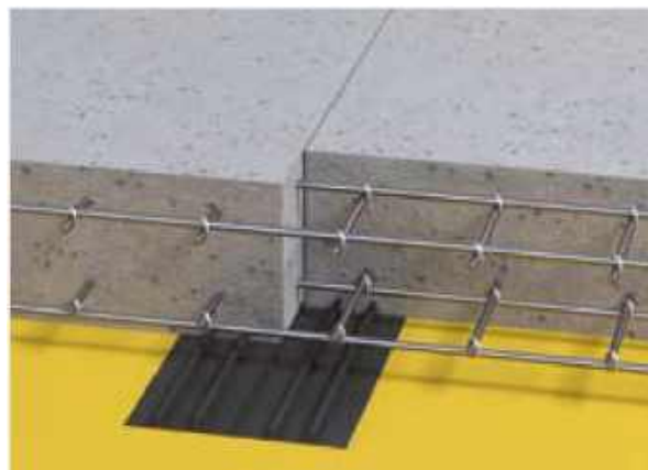
Рисунок 2. Приклад конструктивного рішення застосування зовнішньої гідрошпонки для герметизації швів у монолітних конструкціях
