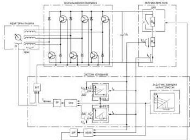
Рисунок.2. Принципова схема автономного вентиляльно-індукторного зварювального генератора
