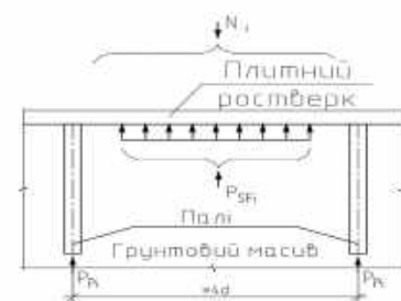
Рисунок. 1 Плитний ростверк
