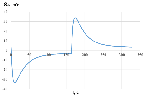
Рисунок 2. Осцилограма термо-ЕРС ТЕМ М2.
