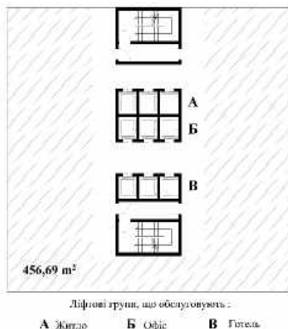
Рис. 1 Схема типового поверху БФК
