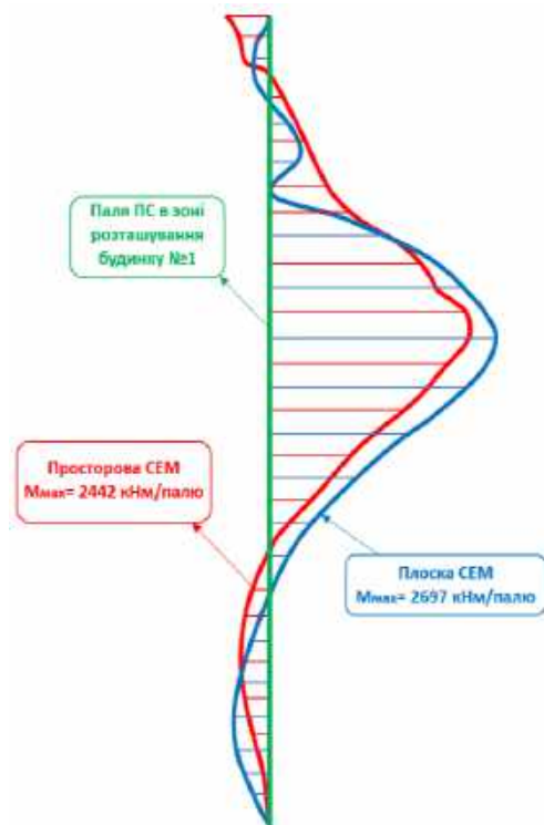
Рисунок 4. Порівняння значень згинальних моментів підпірних стін для кожного з варіантів.
