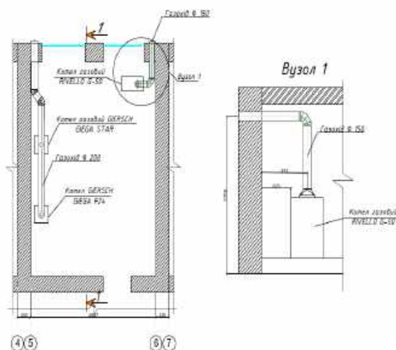
Рисунок 3. Схема димовидалення
