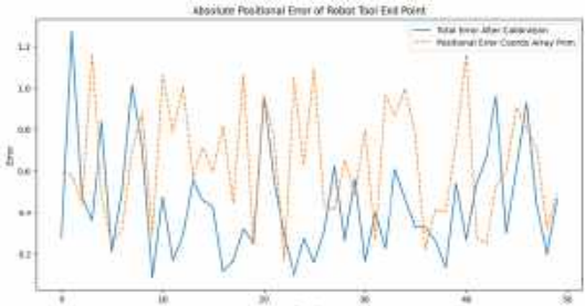
Рис. 3.8 Графік абсолютної позиційної помилки функціональної кінцівки робота маніпулятора
