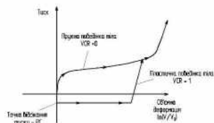
Рисунок 1. Залежність тиску від зміни об'єму для матеріалу ґрунт та піна
