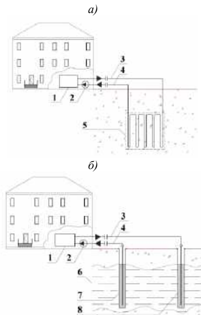
Рисунок 1. Система геотермального охолодження з використанням: а) свердловин; б) водоносного горизонту: 1 – холодильна машина в СКП; 2 – циркуляційний насос; 3 – трубопровід для повернення холодоносія; 4 – трубопровід для підведення холодоносія; 5 – система свердловин; 6 – водоносний горизонт; 7 – видобувна свердловина; 8 – закачувальна свердловина.
