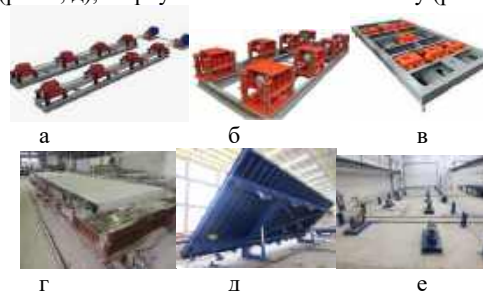
Рисунок 1. Вібраційні машини різних конструкцій
