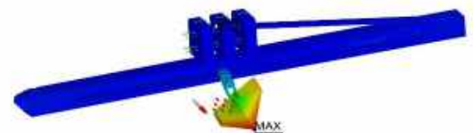
Рисунок 7. Деформації ножа
