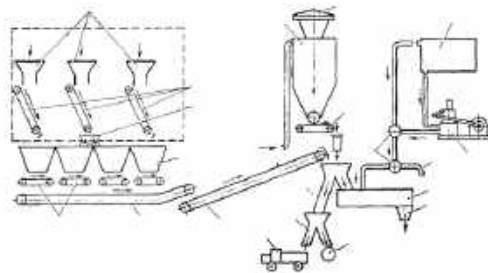
Рисунок 4. Логістична схема бетонозмішувальної установки безперервної дії
