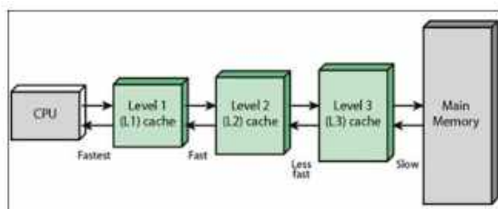
Рисунок 3. Кеш процесора
