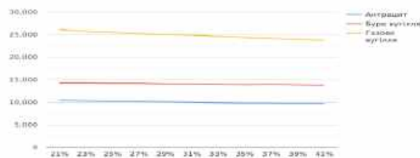
Рисунок 5. Питома витрата палива при різних концентраціях кисню у дуттьовому повітрі, кг/год
