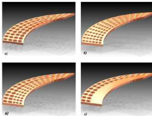
Рисунок 3. Перфоровані гвинтоподібні лопаті, що встановлюються на внутрішній стінці корпусу змішувача по спіралі:
