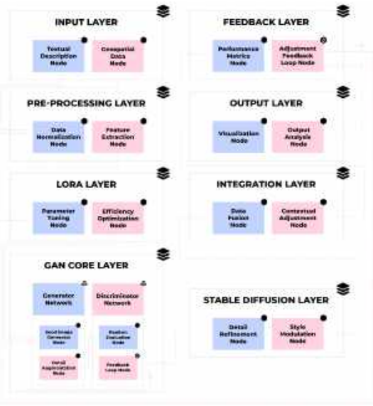
Рисунок 1. Модель інтеграції технології LoRa в GAN Stable Diffusion
