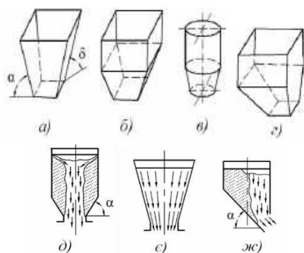
Рисунок 1. Схеми бункерів для перевантаження матеріалів.
