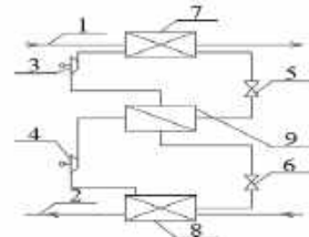
Рисунок 2. Схема підключення здвоєних теплових насосів: 1 – подавальний трубопровід теплової мережі; 2 – зворотний трубопровід теплової мережі; 3 – компресор першого ступеня теплового насосу; 4 – компресор другого ступеня; 5 - дросель-кран першого ступеня теплового насосу; 6 - дросель-кран другого ступеня теплового насосу; 7 – конденсатор; 8 - випарник; 9 – теплообмінник.
