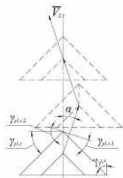
Рисунок 3. План переміщення просторово орієнтованого ножа: при куті \alpha < 45^\circ
