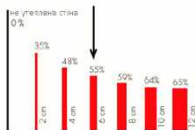
Рисунок 1. Графік залежності тепловтрат в зовнішніх стінах від товщини утеплювача.
