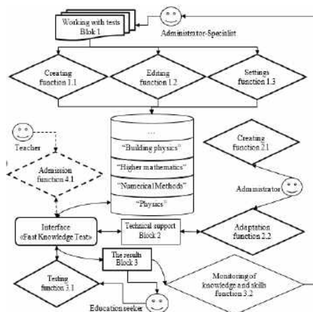
Рисунок 1. Архітектура «Fast Knowledge Test»
