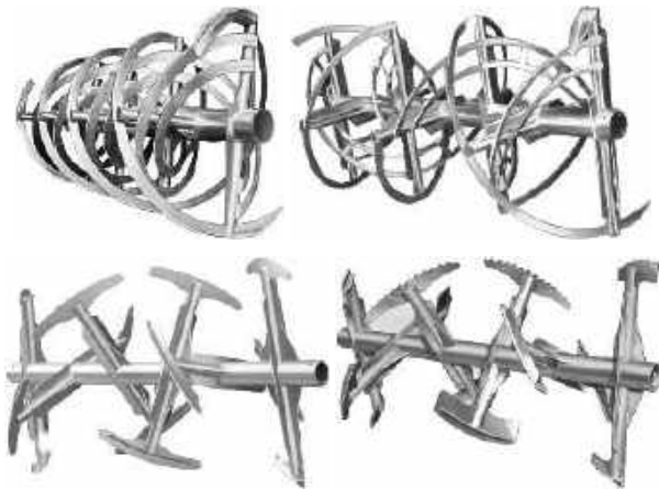
Рисунок 2. Конструкції робочих органів змішувачів сухих будівельних сумішей
