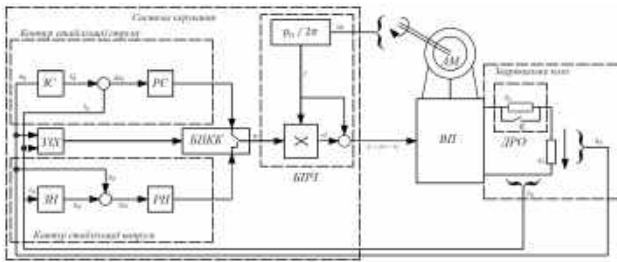
Рисунок.1 Функціональна схема зварювального АГ з ВЗ
