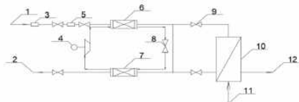
Рисунок 1. Схема теплового насосу в індивідуальному тепловому пункті: 1 – подавальний трубопровід теплової мережі; 2 – зворотний трубопровід теплової мережі; 3 – відмулювач; 4 – компресор; 5 – сітчастий фільтр; 6 – конденсатор; 7 – випарник; 8 – дросель-кран; 9 – запірні арматури; 10 – пластинчастий теплообмінник; 11 – зворотний трубопровід від споживача; 12 – подавальний трубопровід до споживача.
