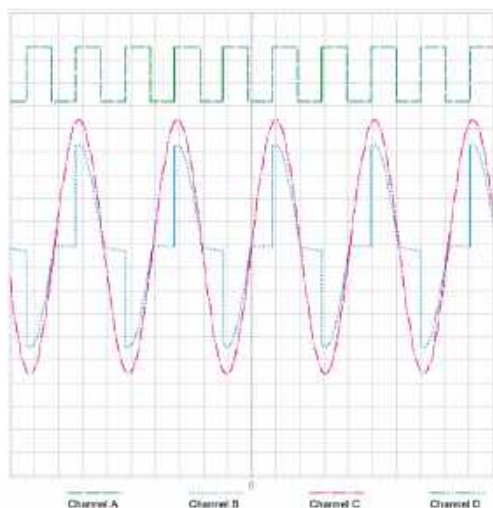
Рисунок 3. Осцилограма роботи модуля при 50% заповненні ШІМ
