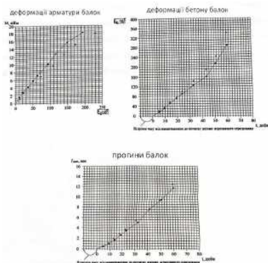
Рисунок 2. Деформації арматури, бетону балок та прогини балок.
