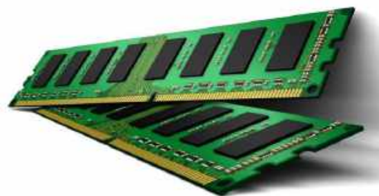
Рисунок 1. Оперативна пам'ять(RAM)
