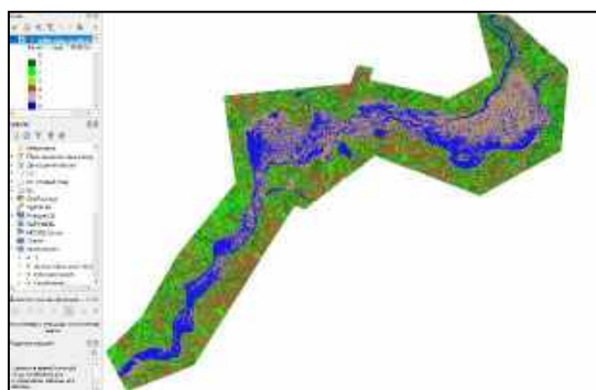
Рисунок 2. Класифікований космічний знімок супутника Sentinel-2 L2 у середовищі QGIS
