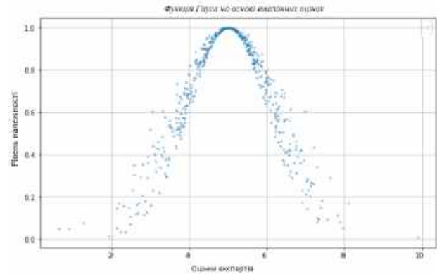
2. Рисунок 3. Функція Гауса для визначення рівня належності оцінки експерта
