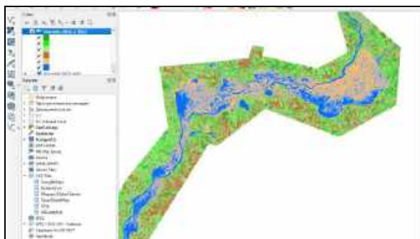
Рисунок 2. Класифікований космічний знімок супутника Sentinel-2 L2 у середовищі QGIS
