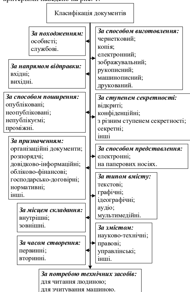
Рисунок 1. Класифікація документів
