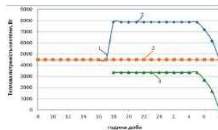
Рисунок 2. Зміни теплової потужності протягом доби систем нікелювального відділення: 1, 2 комбінованої в робочий (8-17 години) та черговий (18-24-8 години) використання приміщення; 3 – фонові; – догрівачої
