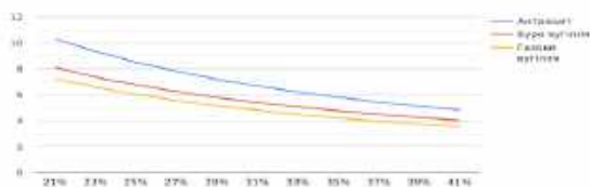
Рисунок 3. Об'єм продуктів горіння при різних концентраціях кисню у дуттьовому повітрі, м 3 /кг [1]
